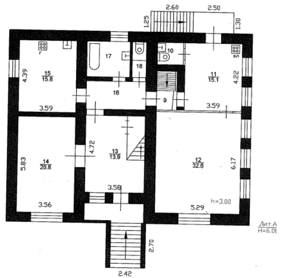
1 этаж
