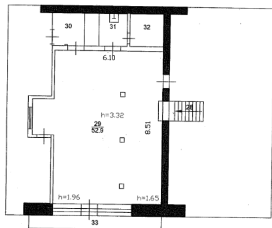
Мансардный этаж
