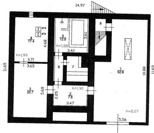
Цокольный этаж
