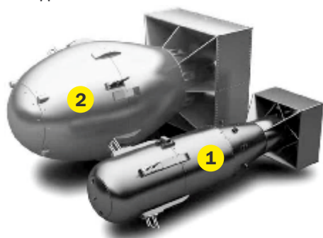
1 «Little Boy» (Малыш): диаметр – 70 см, длина – 3 м, масса – 4 400 кг.
